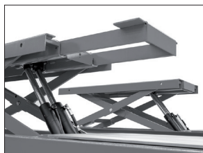
Chemins avec double levage + extensible.
