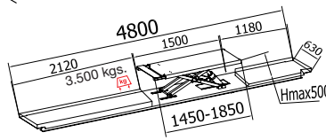
Pasarela lisa con elevación auxiliar hidráulica.
