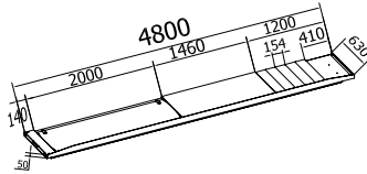
Pasarela de alineación .
