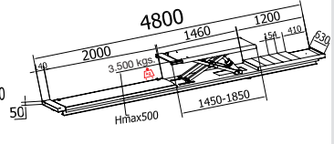
Pasarela de alineación con elevación auxiliar hidráulica.
